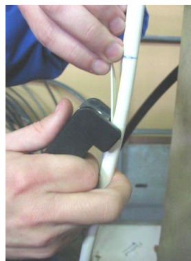
② Ouverture d'un câble distribution intérieur (Exemple d'application)
